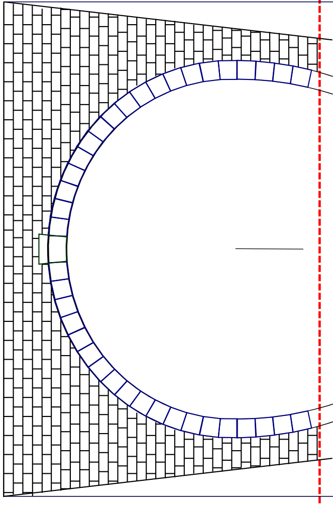
Portale doppio - rettilineo - linea aerea
