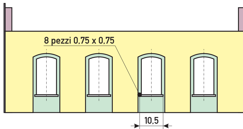
vista laterale
